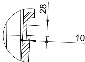
C (1 : 5)
