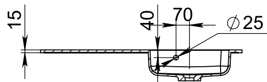
A-A
